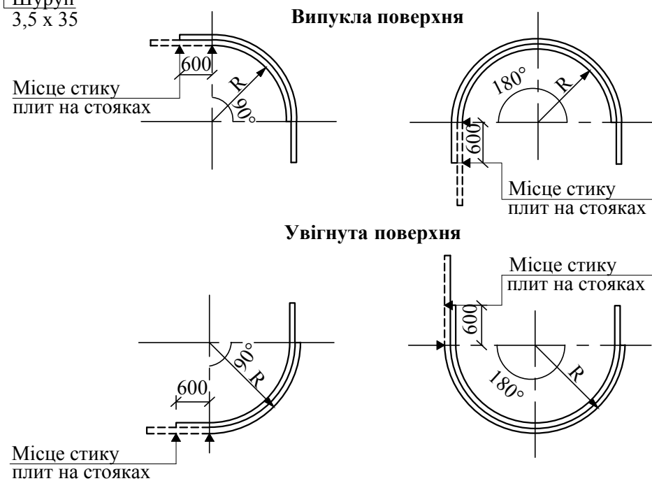
Схема місць стику плит при двохшаровій обшивці на початку і в кінці криволінійної ділянки
