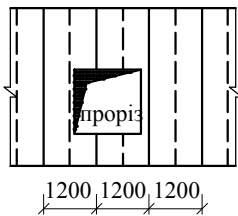
Розташування 2-го шару ГКП
