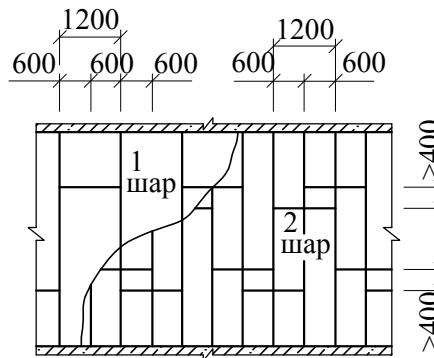
Розташування плит гіпсокартону при одношаровій та двошаровій обшивці каркаса
