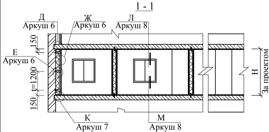
Розташування плит гіпсокартону при одношаровій та двошаровій обшивці каркаса
