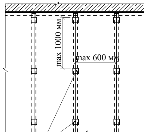
З'єднувач віброакустичний Siniat PWA 50 встановлюється з кроком менше 1000 мм x 600 мм
